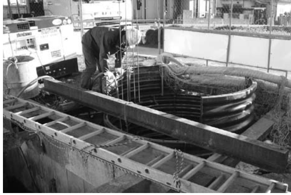
污水管損傷の復旧工事
