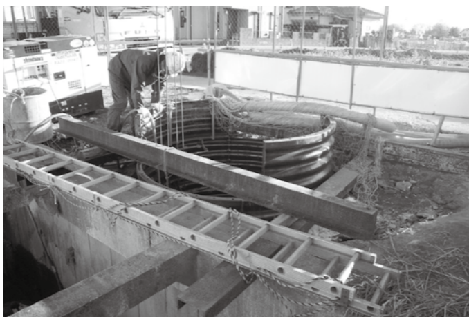
汚水管損傷の復旧工事
